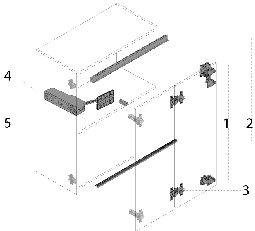
Vista general del sistema
